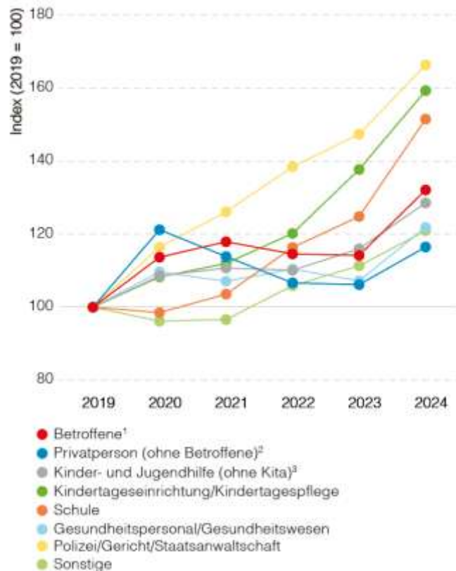
Abb. 3: Indexentwicklung der 8a-Verfahren nach Hinweisgebenden (Deutschland; 2019 bis 2024; Index 2019 = 100)
